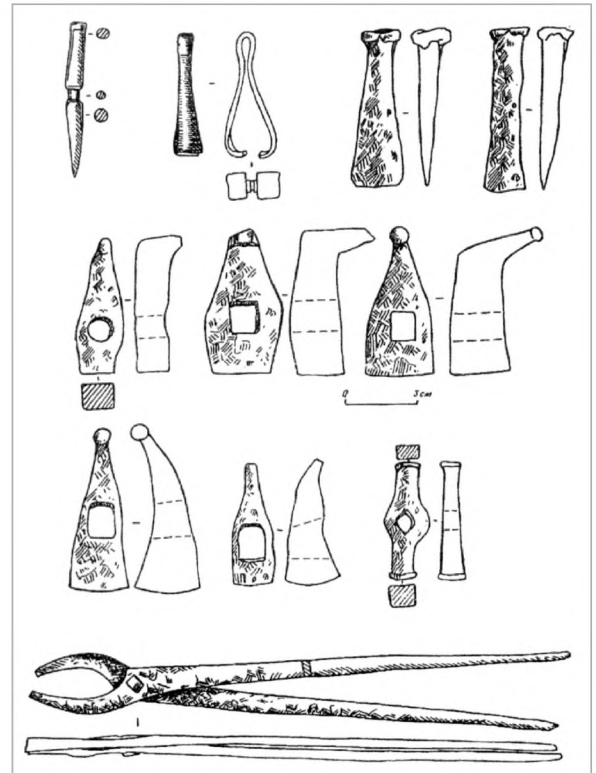
Инструментарий кузнецов и ювелиров
