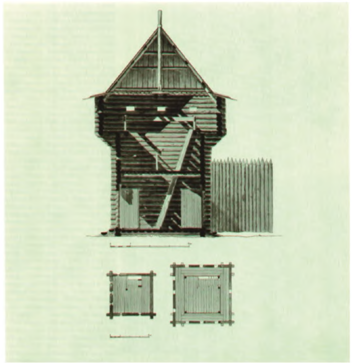
Проездная башня. Фасад, план. Разрез плана разных ярусов. Реконструкция
